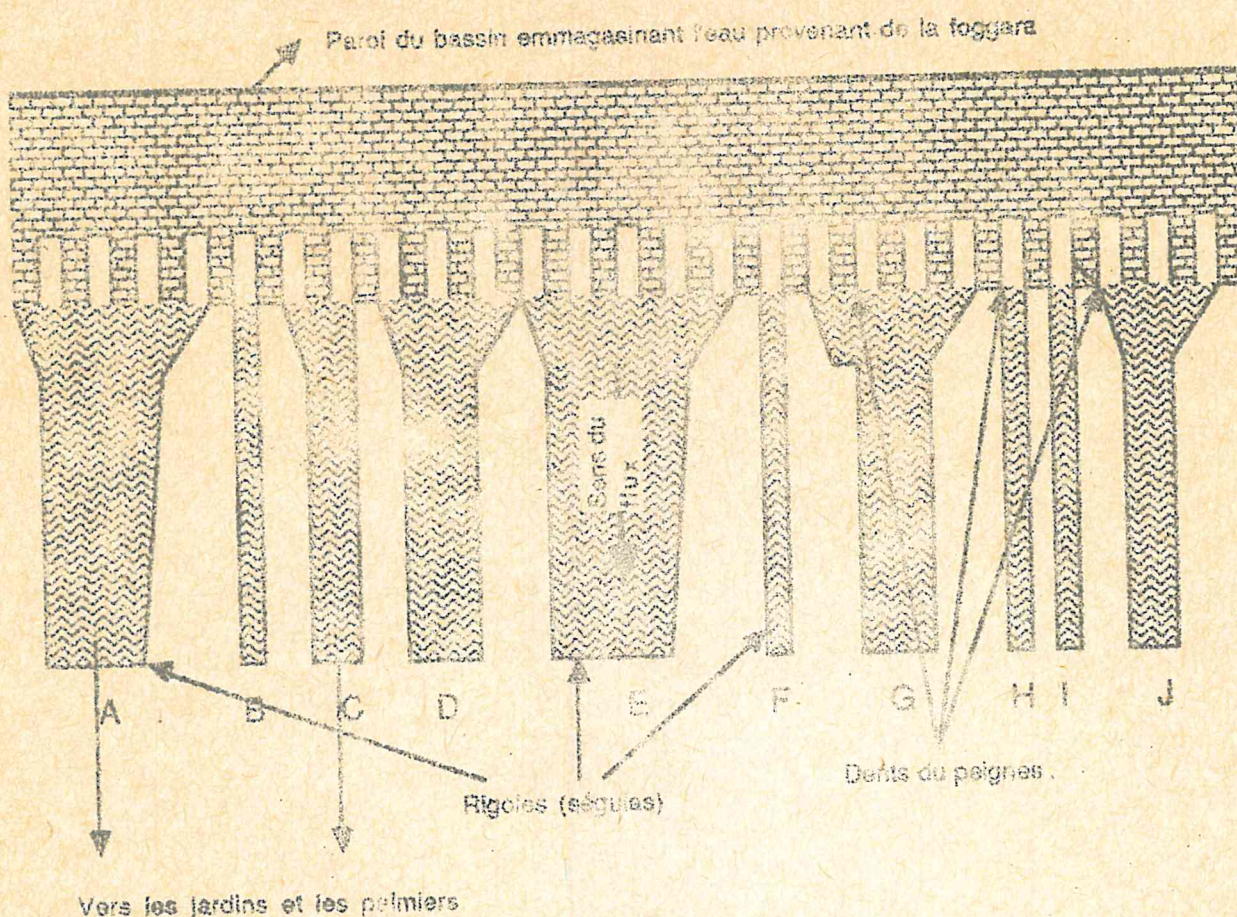
Schéma d'un peigne de foggara
